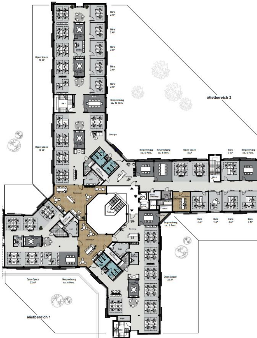
2.OG Regelgeschoss mit MB 1 und MB 2
